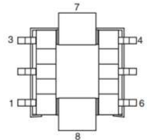
底视图
