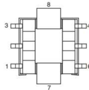
底视图
